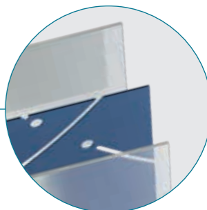
VITRAGE DESIGN COMPOSÉ DE : 1 DOUBLE VITRAGE FEUILLETÉ 44/6 CLAIR CÔTÉ EXTÉRIEUR. 1 TÔLE ALUMINIUM THERMOLAQUÉE DÉCOR DESIGN 1 DOUBLE VITRAGE FEUILLETÉ 44/6 DÉPOLI ACIDE CÔTÉ INTÉRIEUR
